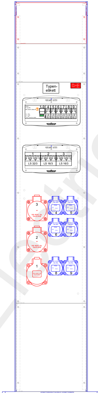
Ansicht geschlossen
